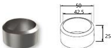
Wall cover for column Ø42 Κωδ. / Code 4510 Συσκ. / Pack. 50 τεμ./pcs.
