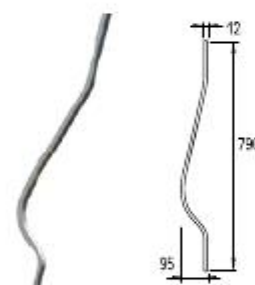
Curved profile for Vertical-D Κωδ. / Code 4680 Συσκ. / Pack. 100 τεμ./pcs.
