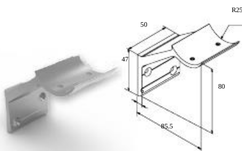
Support foot for Ø42 column Κωδ. / Code 4126 Συσκ. / Pack. 20 τεμ./pcs.
