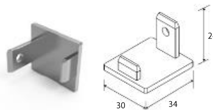
End cap for F50-319 guide Κωδ. / Code 4477 Συσκ. / Pack. 40 τεμ./pcs.
