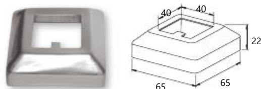
Wall cover for F50-102 column Κωδ. / Code 4514 Συσκ. / Pack. 50 τεμ./pcs.
