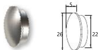
End cap for F50-304 profile Κωδ. / Code 4461 Συσκ. / Pack. 50 τεμ./pcs.
