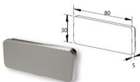
End cap for F50-201 handrail Κωδ. / Code 4447 Συσκ. / Pack. 20 τεμ./pcs.
