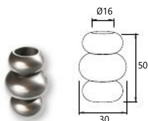
Glass rosette for profile Ø16 Κωδ. / Code 4618 Συσκ. / Pack. 50 τεμ./pcs.
