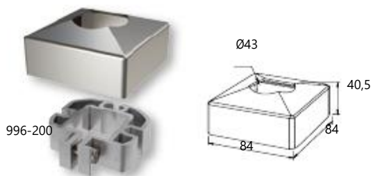
Support foot for Ø42 column Κωδ. / Code 4126 Συσκ. / Pack. 20 τεμ./pcs.
