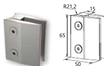
Glass support 8-10 mm Κωδ. / Code 4168 Συσκ. / Pack. 50 τεμ./pcs.
