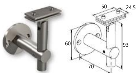
F50-201 Railtop wall support Κωδ. / Code F85-452 Συσκ. / Pack. 40 τεμ./pcs.
