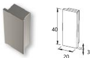
End cap for 59-009 profile Κωδ. / Code 4464 Συσκ. / Pack. 50 τεμ./pcs.
