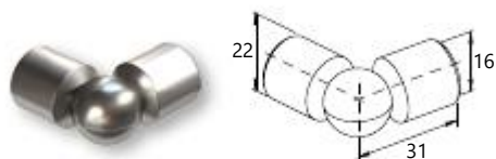
Adjustable angle connector for profile Ø16 Κωδ. / Code 4302 Συσκ. / Pack. 50 τεμ./pcs.
