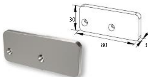
End cap for F50-203 handrail Κωδ. / Code 4451 Συσκ. / Pack. 10 ζευγ./pair
