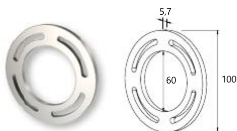
Glass rosette Ø100 Κωδ. / Code 4611 Συσκ. / Pack. 20 τεμ./pcs.
