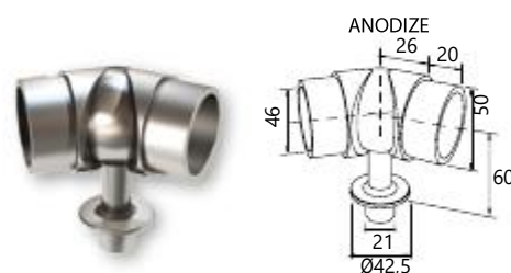
Connector for F50-100 column with guide Ø16 Κωδ. / Code 4312 Συσκ. / Pack. 12 τεμ./pcs.
