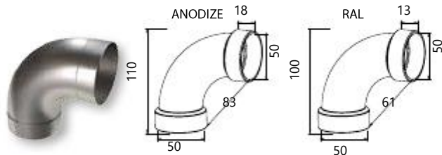
κουπαστών Ø50 Connector 90° for handrail Ø50 Κωδ. / Code 4219 Συσκ. / Pack. 20 τεμ./pcs.
