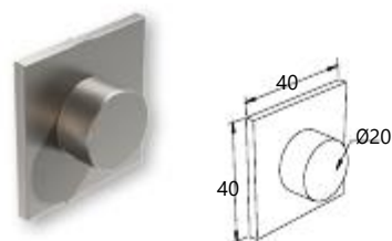
End cap for F50-102 column Κωδ. / Code 4448 Συσκ. / Pack. 40 τεμ./pcs.
