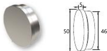
End cap for F50-200 handrail (flat) Κωδ. / Code 4453 Συσκ. / Pack. 50 τεμ./pcs.
